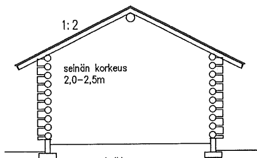
Leikkaus
